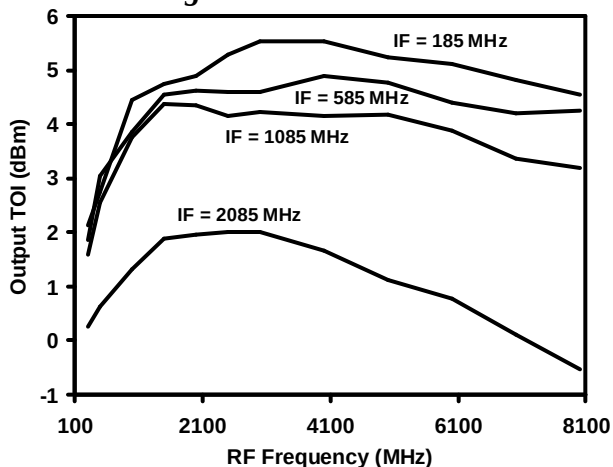
Figure 8. Output TOI.
